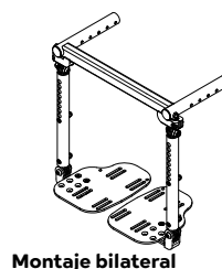
Montaje bilateral
